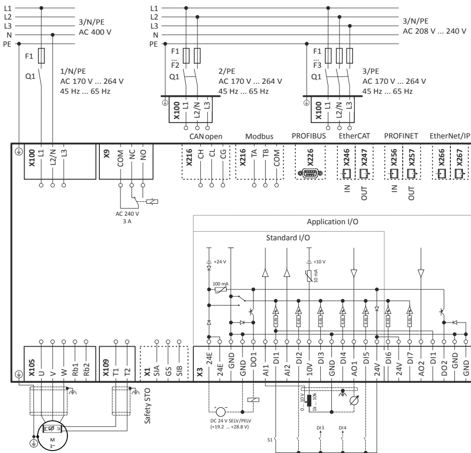
Fig. 2: Wiring example
