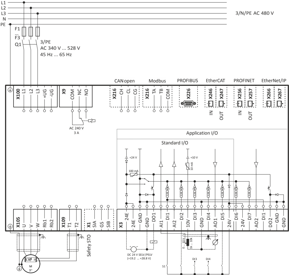
Fig. 3: Wiring example
